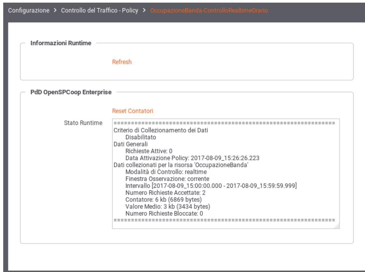
Figure8.67: Dati statistici relativi ad una policy di rate limiting
