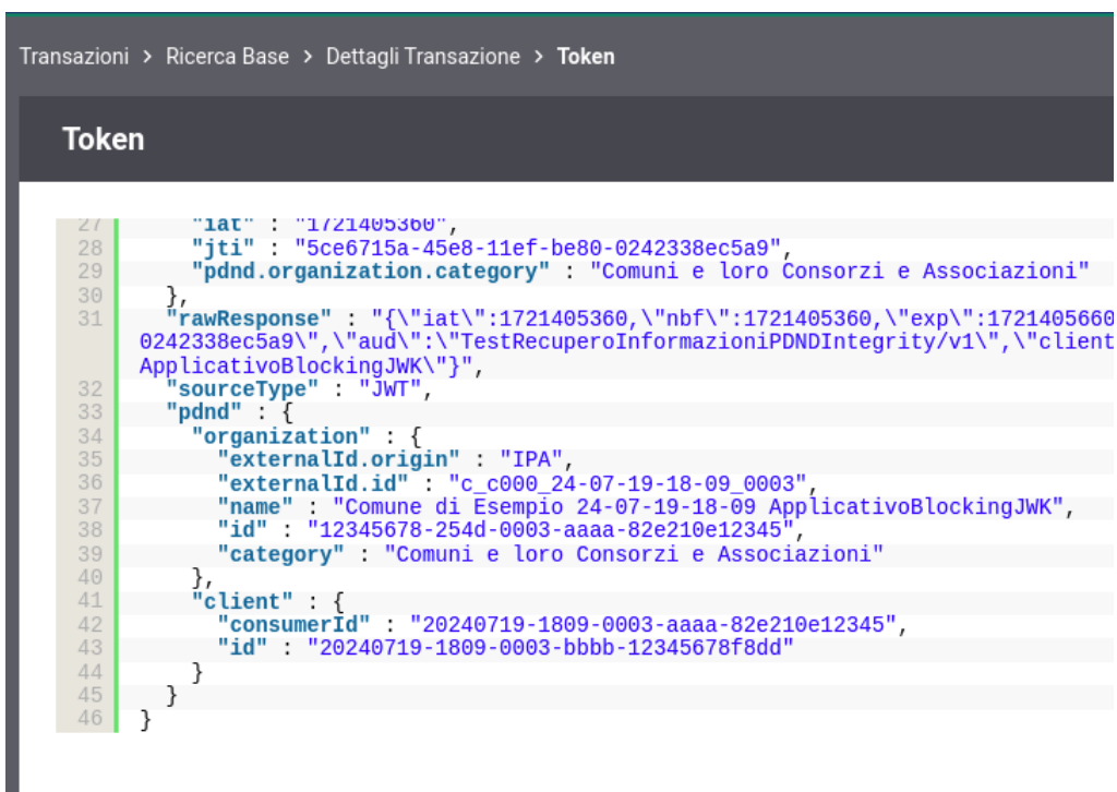
Figure3.146: Informazioni ottenute tramite API PDND
