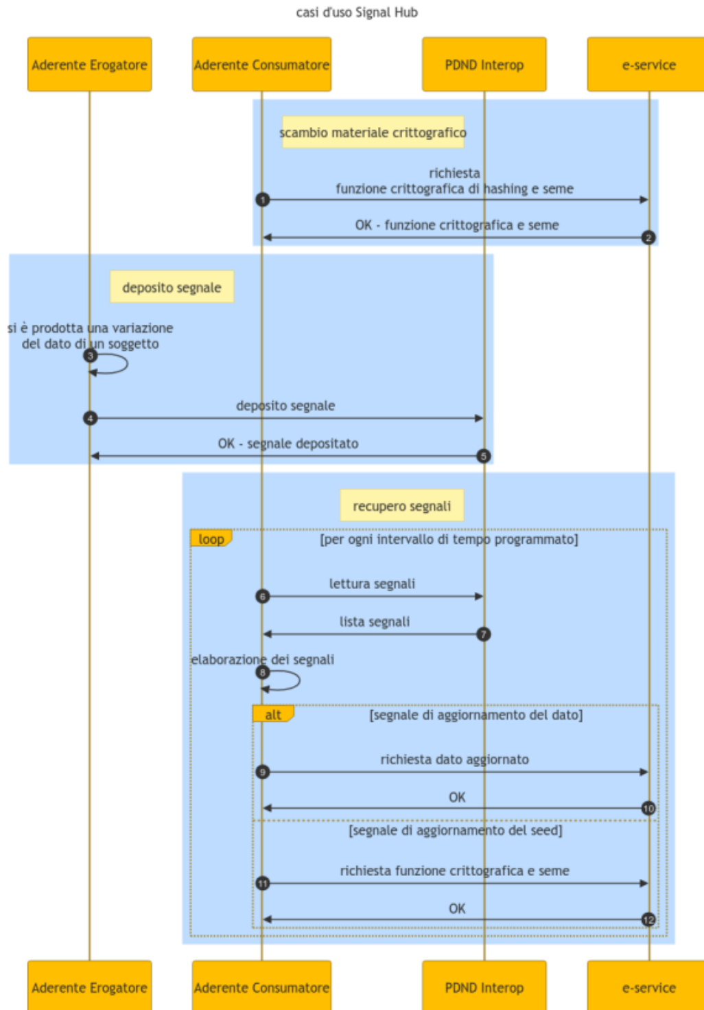
Figure3.174: Diagramma di sequenza per l'utilizzo da parte di un aderente della funzionalità Signal Hub
