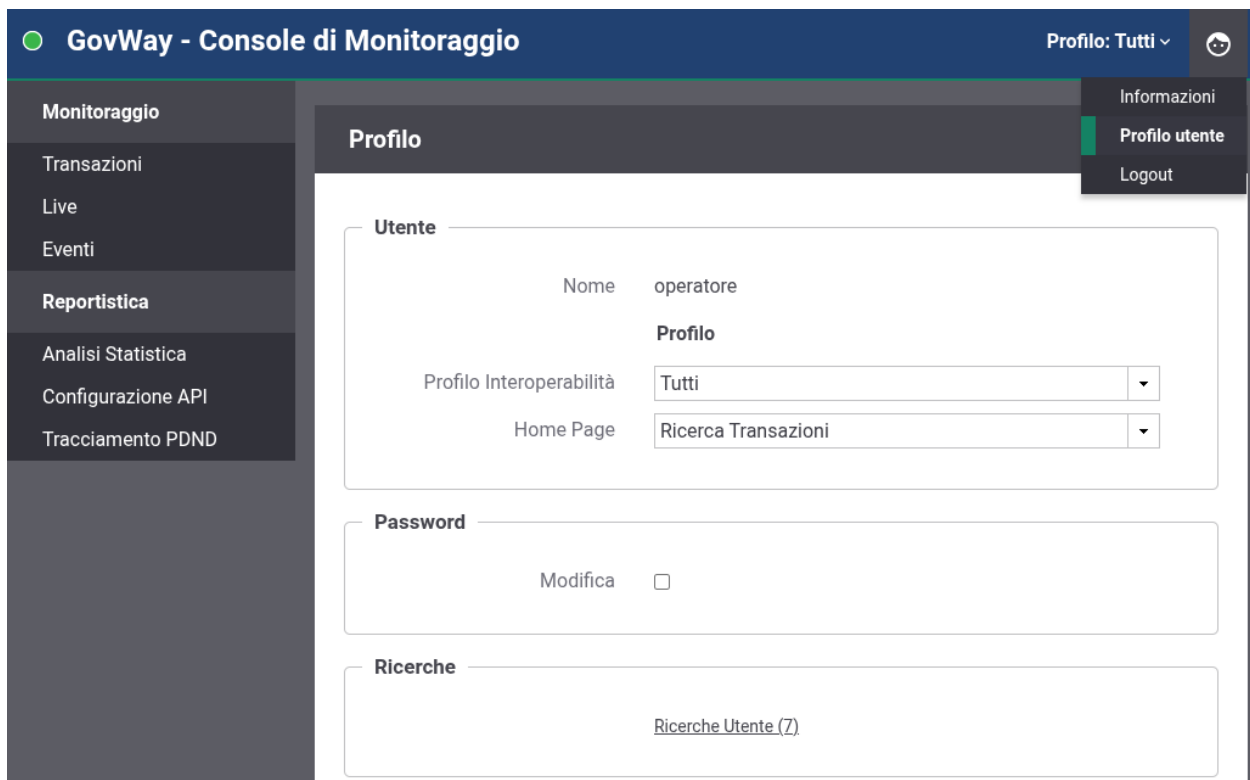
Figure2.9: Profilo Utente
