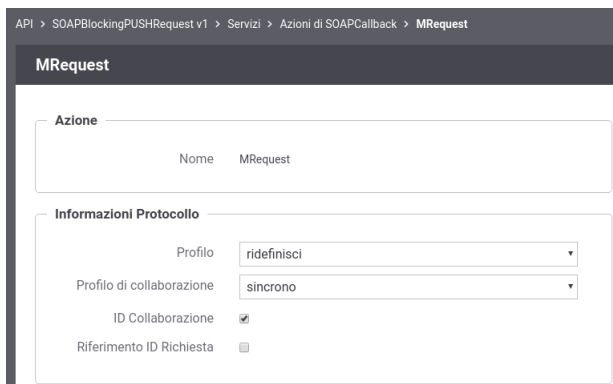
Fig. 3.48: Abilitazione funzionalità di correlazione govway tramite identificativo di collaborazione
