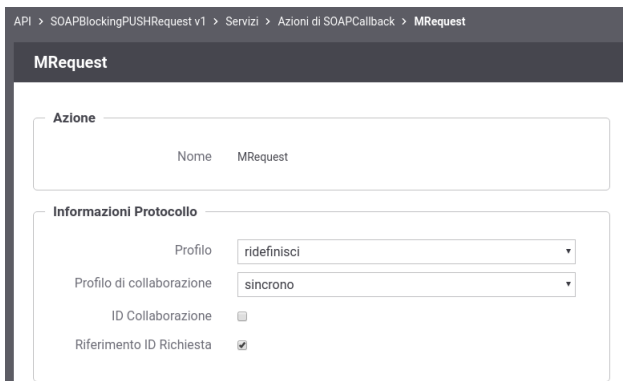
Fig. 3.49: Abilitazione funzionalità di correlazione govway tramite identificativo della richiesta
