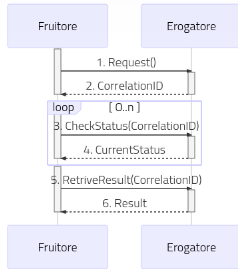
Fig. 3.55: Flusso previsto in un Pattern di Interazione PULL per API SOAP
