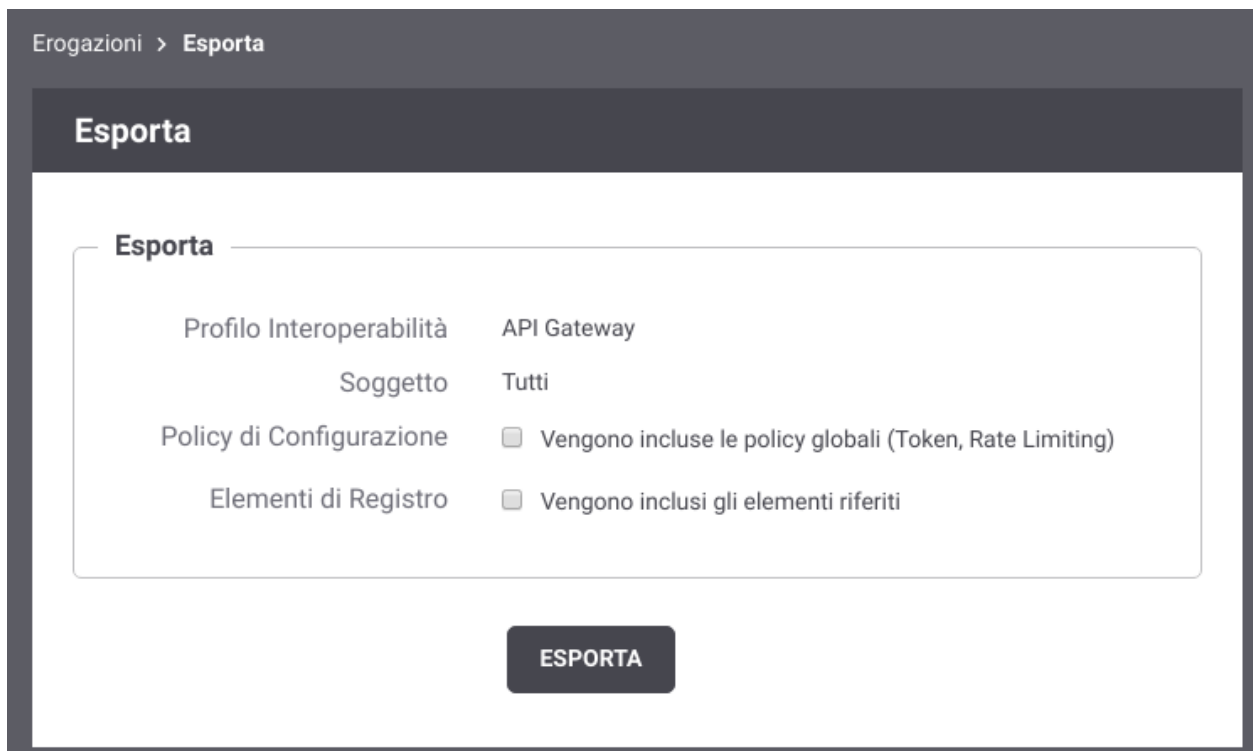
Fig. 8.54: Esportazione di entità nel registro: parametri
