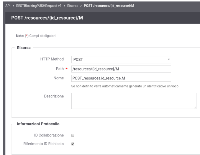
Fig. 3.54: Abilitazione funzionalità di correlazione govway tramite identificativo della richiesta
