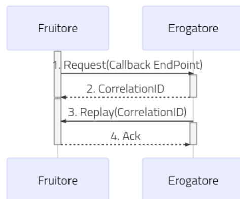
Fig. 3.50: Flusso previsto in un Pattern di Interazione PUSH
