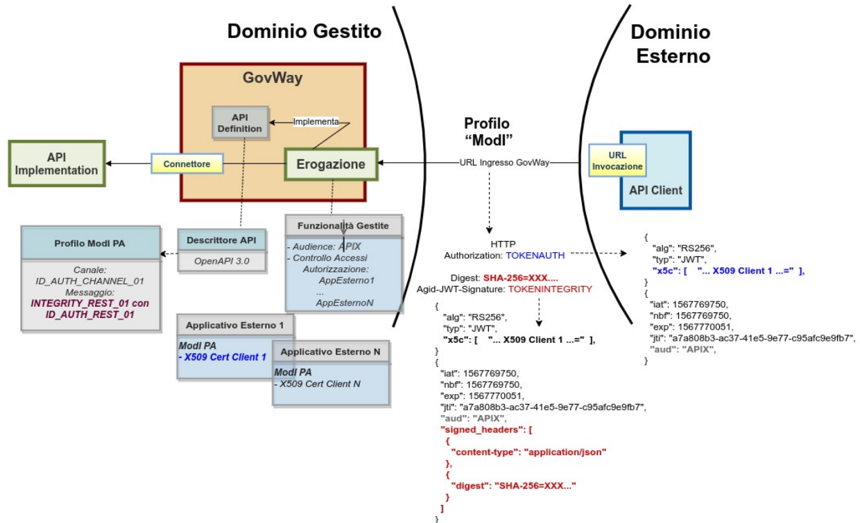
Figure3.88: Erogazione con Profilo di Interoperabilità “Modi”, pattern “INTEGRITY_REST_01”: trust tra fruitore ed erogatore tramite certificati x509
