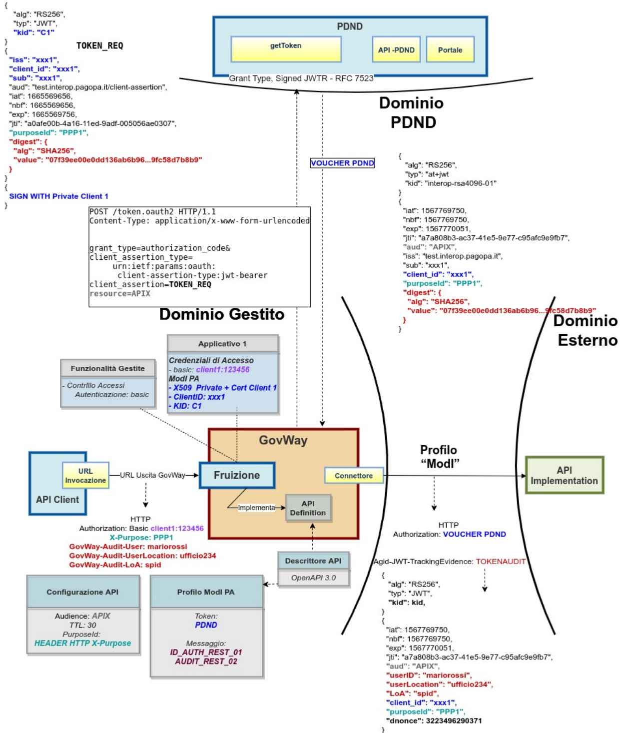
Figure3.103: Profilo di Interoperabilità "ModI", pattern "AUDIT_REST_02": trust tramite PDND
