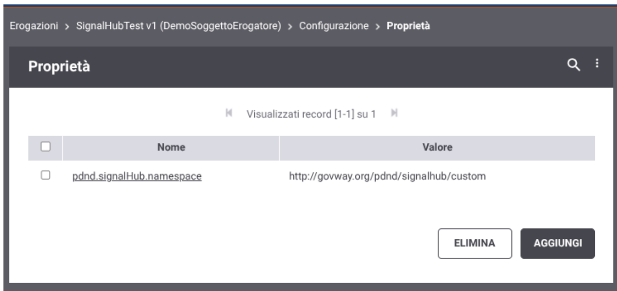
Figure3.173: Schermata di configurazione della proprietà per impostare un namespace personalizzato.
