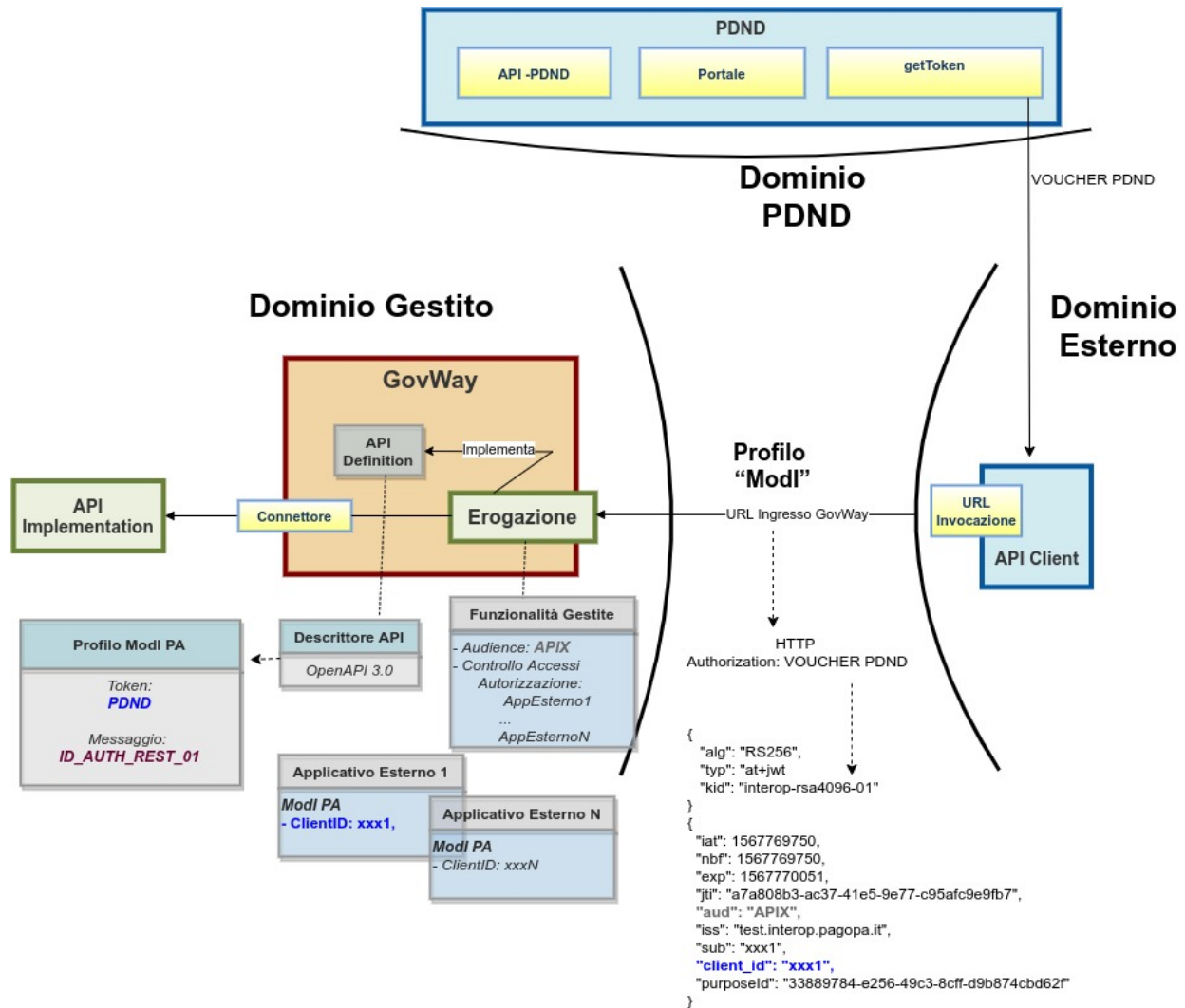
Figure3.41: Erogazione con Profilo di Interoperabilità “ModI”, pattern “ID_AUTH_REST_01”: trust tramite PDND
