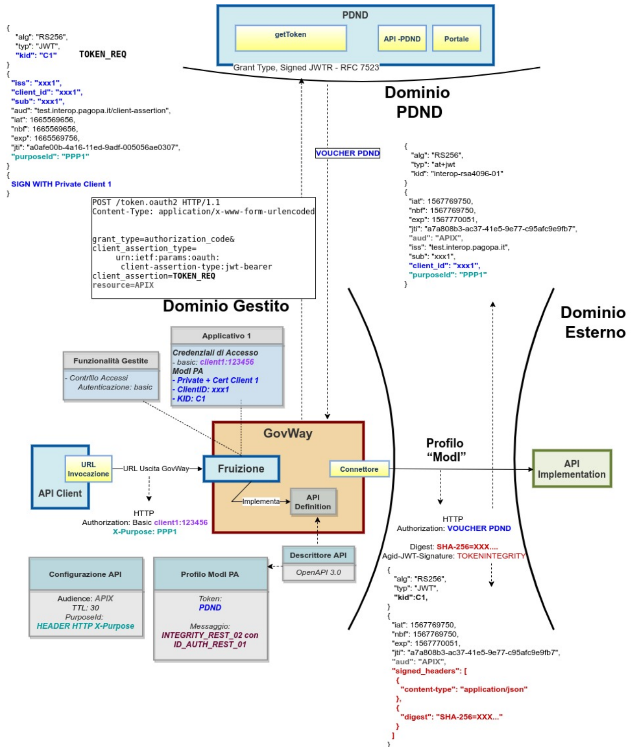
Figure3.73: Fruizione con Profilo di Interoperabilità “Modi”, pattern “INTEGRITY_REST_02”: trust tramite PDND
