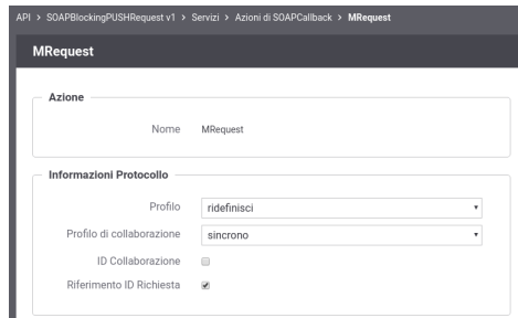
Figure3.151: Abilitazione funzionalità di correlazione govway tramite identificativo della richiesta
