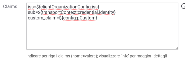
Figure3.129: Claims aggiuntivi inseriti nel Payload JWT
