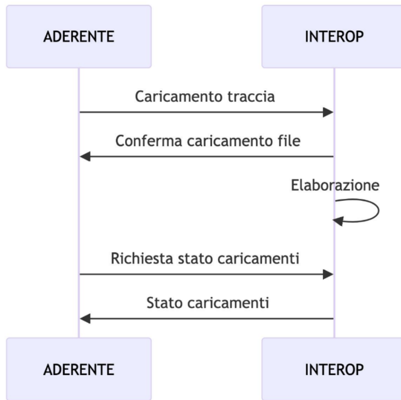
Figure3.180: Diagramma di sequenza della fase di pubblicazione del tracciato e recupero asincrono dello stato
