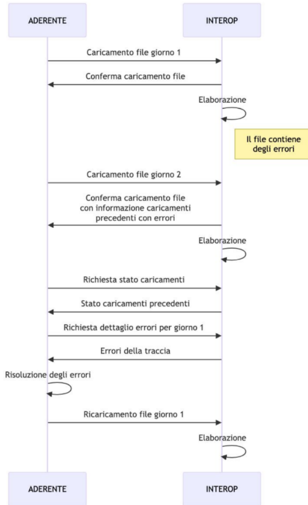
Figure3.181: Sostituzione di un tracciato caricato contenente errori.
