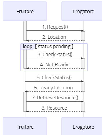
Figure3.163: Flusso previsto in un Pattern di Interazione PULL per API REST
