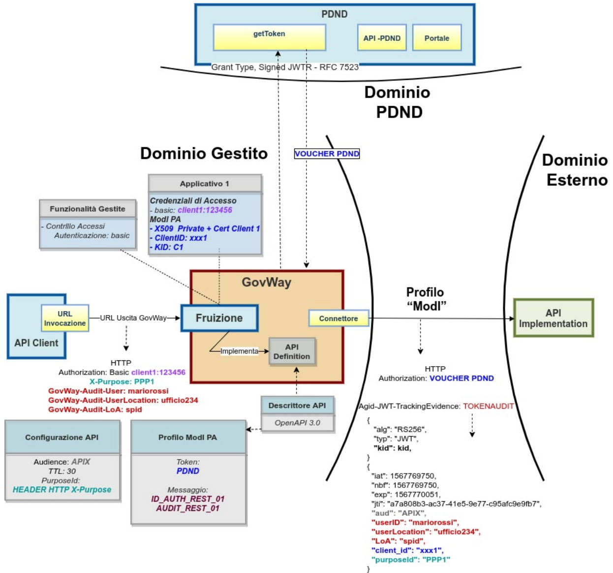
Figure3.98: Fruizione con Profilo di Interoperabilità “Modi”, pattern “AUDIT_REST_01”: trust tramite PDND
