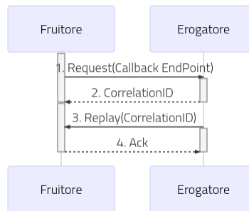
Figure3.147: Flusso previsto in un Pattern di Interazione PUSH
