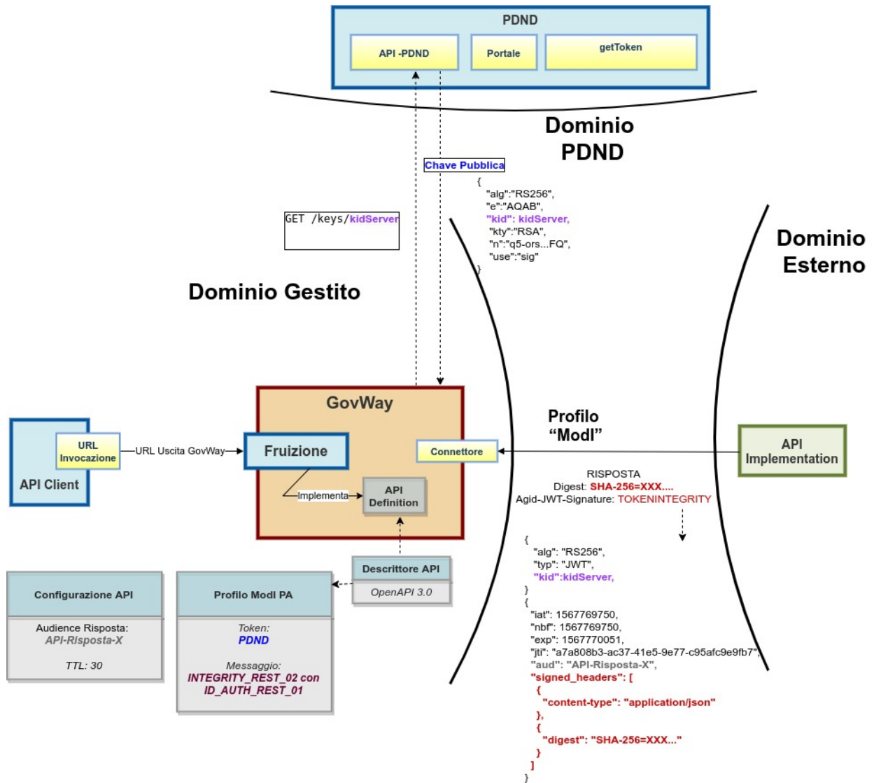
Figure3.78: Fruizione con Profilo di Interoperabilità “ModI”, pattern “INTEGRITY_REST_02”: trust tramite PDND e utilizzo delle API PDND per ottenere la chiave pubblica per validare la risposta
