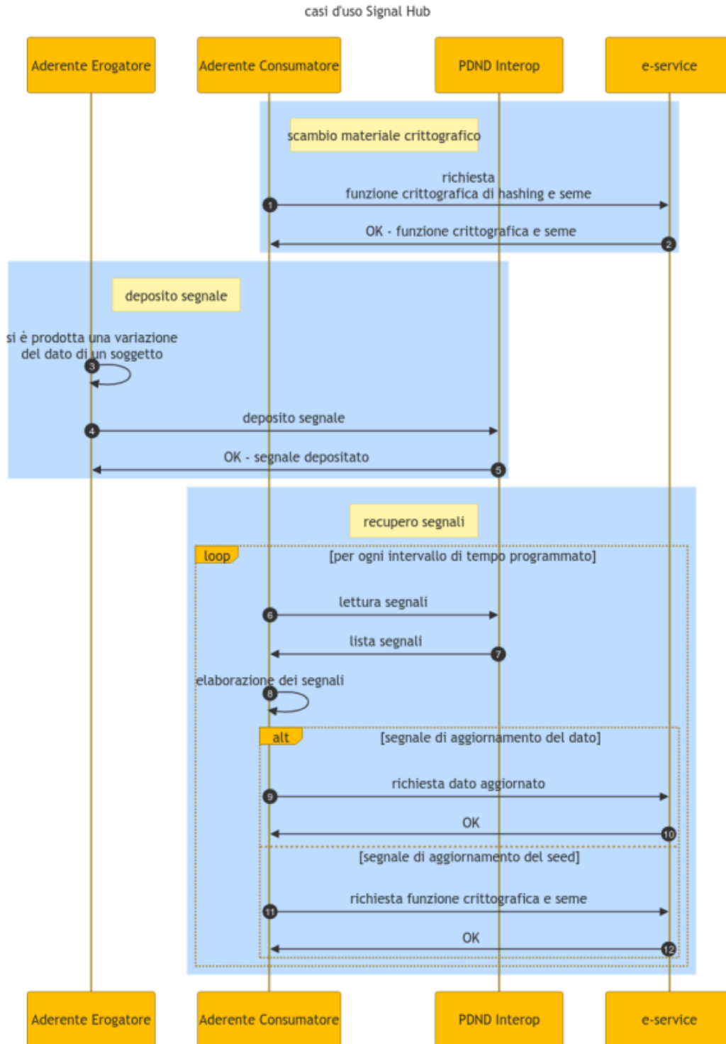
Figure3.168: Diagramma di sequenza per l'utilizzo da parte di un aderente della funzionalità Signal Hub
