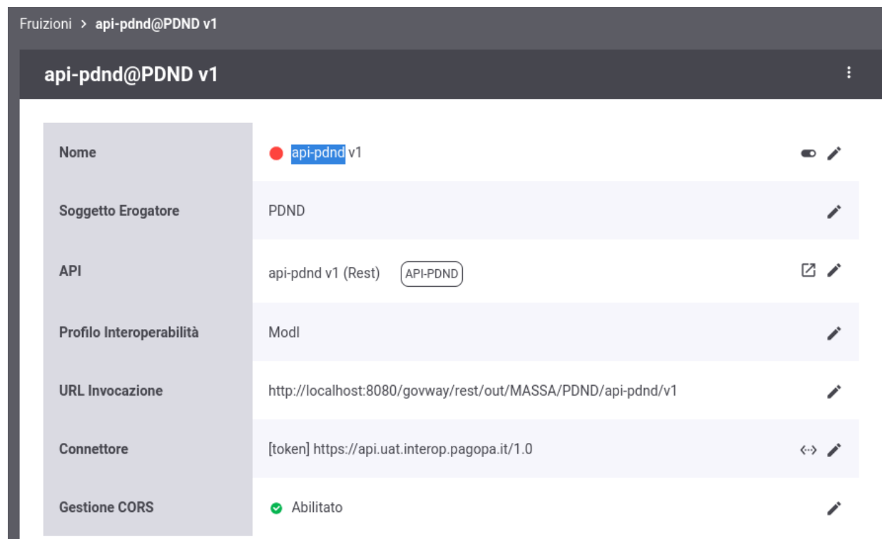
Figure3.14: Fruizione delle API PDND
