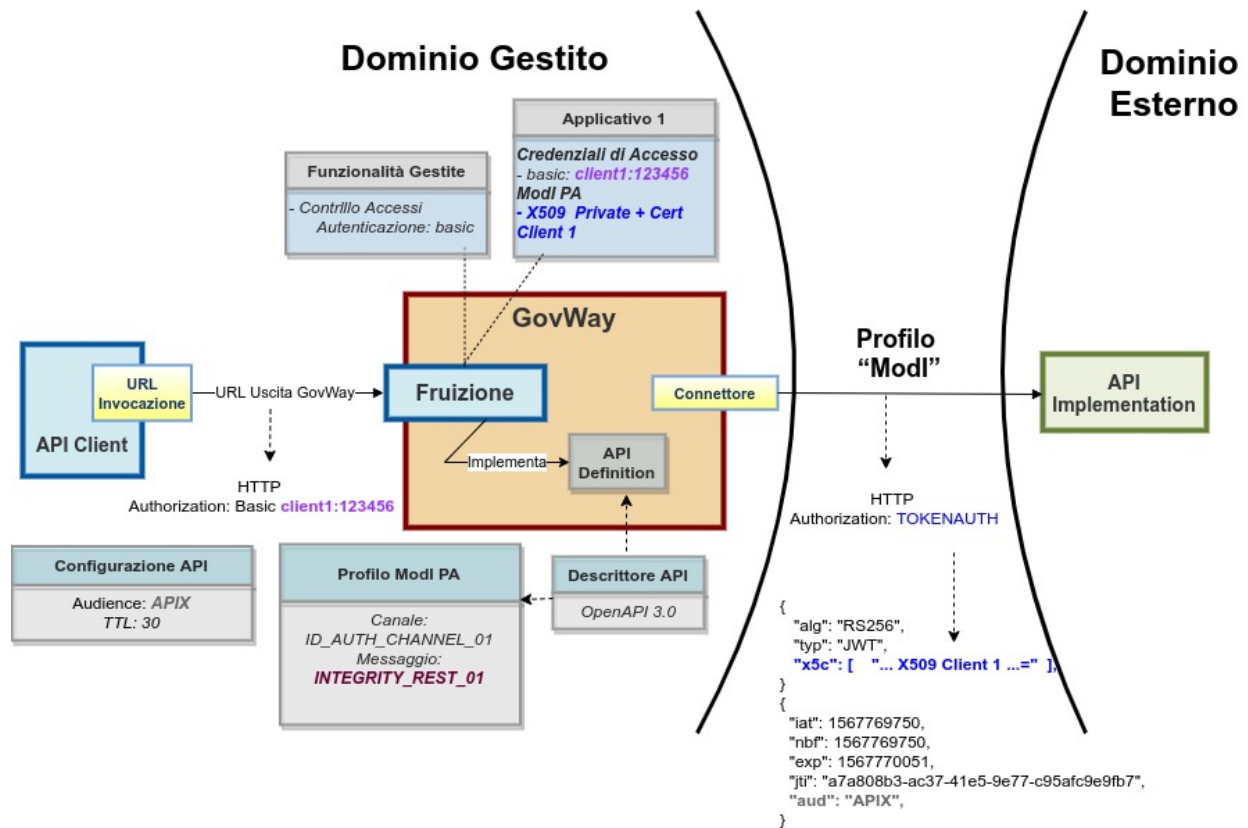
Figure3.54: Fruizione con Profilo di Interoperabilità “ModI”, pattern “ID_AUTH_REST_01”: trust tra fruitore ed erogatore tramite certificati x509
