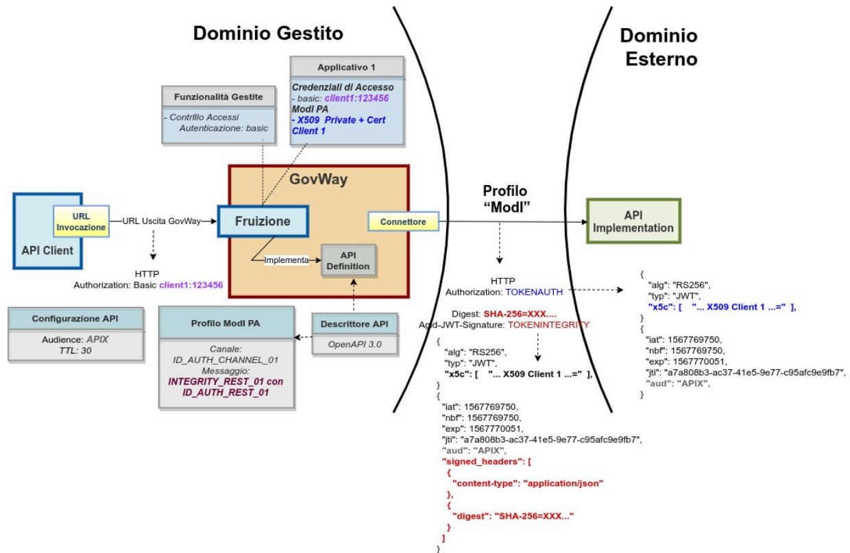
Figure3.86: Fruizione con Profilo di Interoperabilità “ModI”, pattern “INTEGRITY_REST_01”: trust tra fruitore ed erogatore tramite certificati x509
