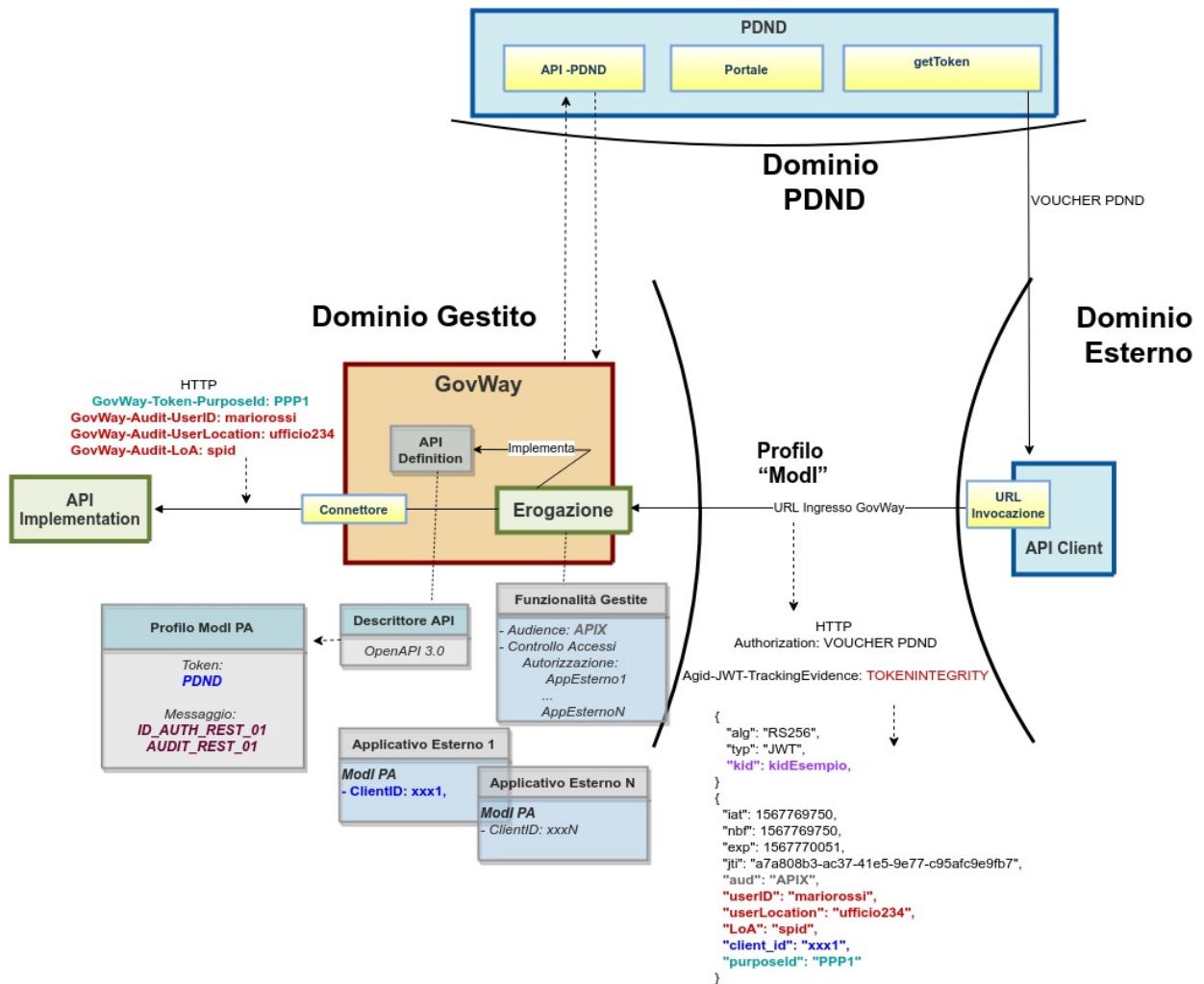
Figure3.101: Erogazione con Profilo di Interoperabilità "Modi", pattern "AUDIT_REST_01": trust tramite PDND
