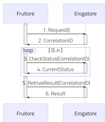
Figure3.157: Flusso previsto in un Pattern di Interazione PULL per API SOAP
