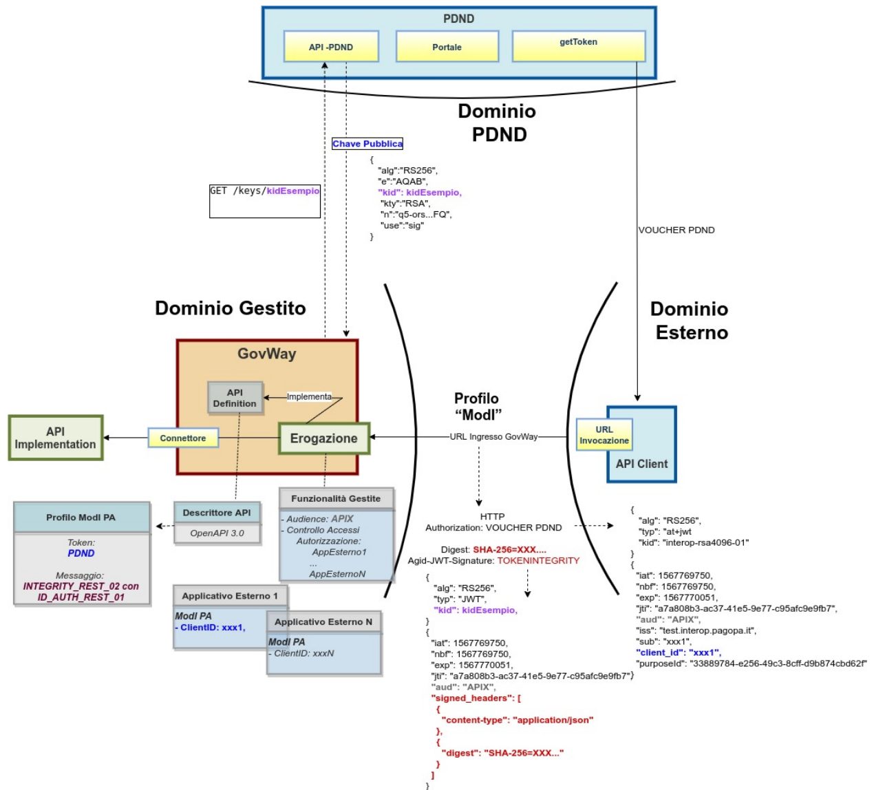
Figure3.79: Erogazione con Profilo di Interoperabilità “ModI”, pattern “INTEGRITY_REST_02”: trust tramite PDND
