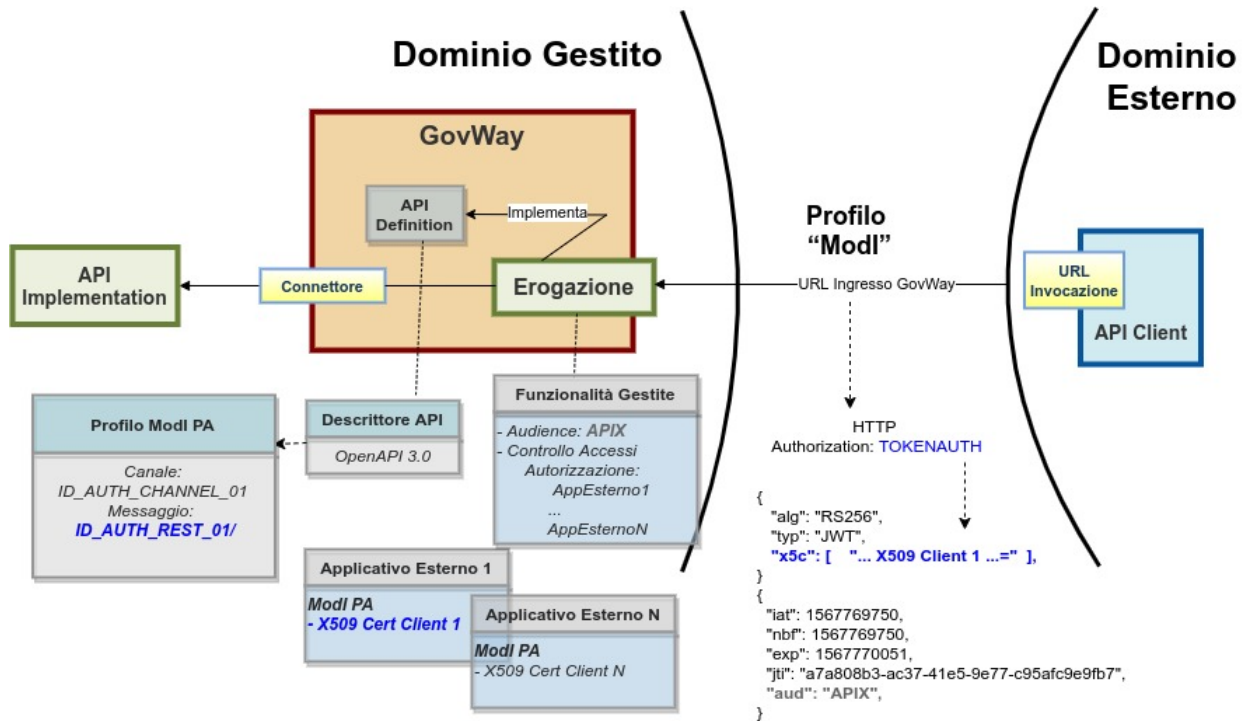
Figure3.58: Erogazione con Profilo di Interoperabilità “ModI”, pattern “ID_AUTH_REST_01”: trust tra fruitore ed erogatore tramite certificati x509
