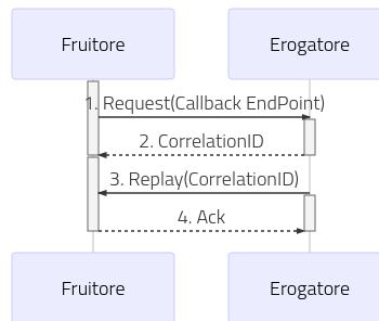
Figure3.152: Flusso previsto in un Pattern di Interazione PUSH
