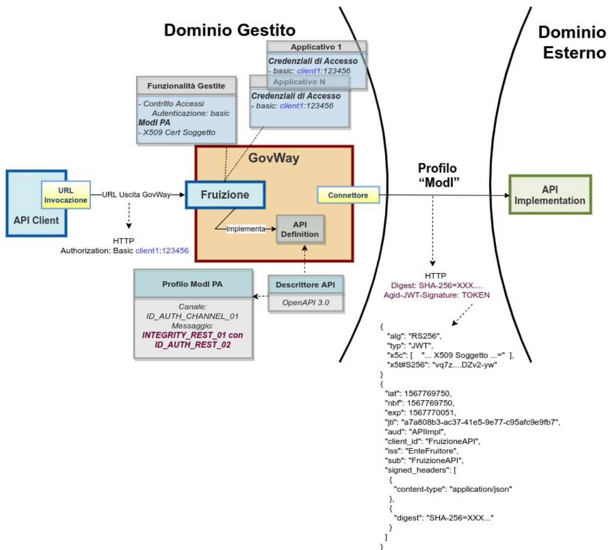
Figure3.133: Fruizione con Profilo di Interoperabilità “ModI”; keystore definito nella fruizione
