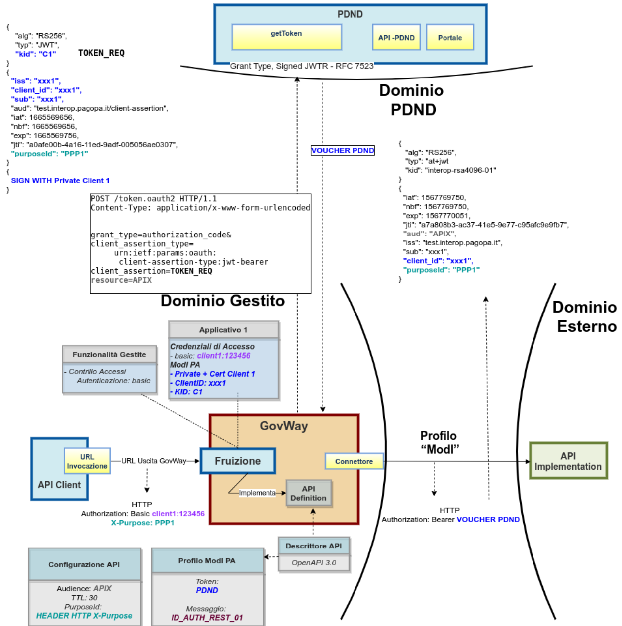
Figure3.18: Fruizione con Profilo di Interoperabilità "ModI", pattern "ID_AUTH_REST_01": trust tramite PDND
