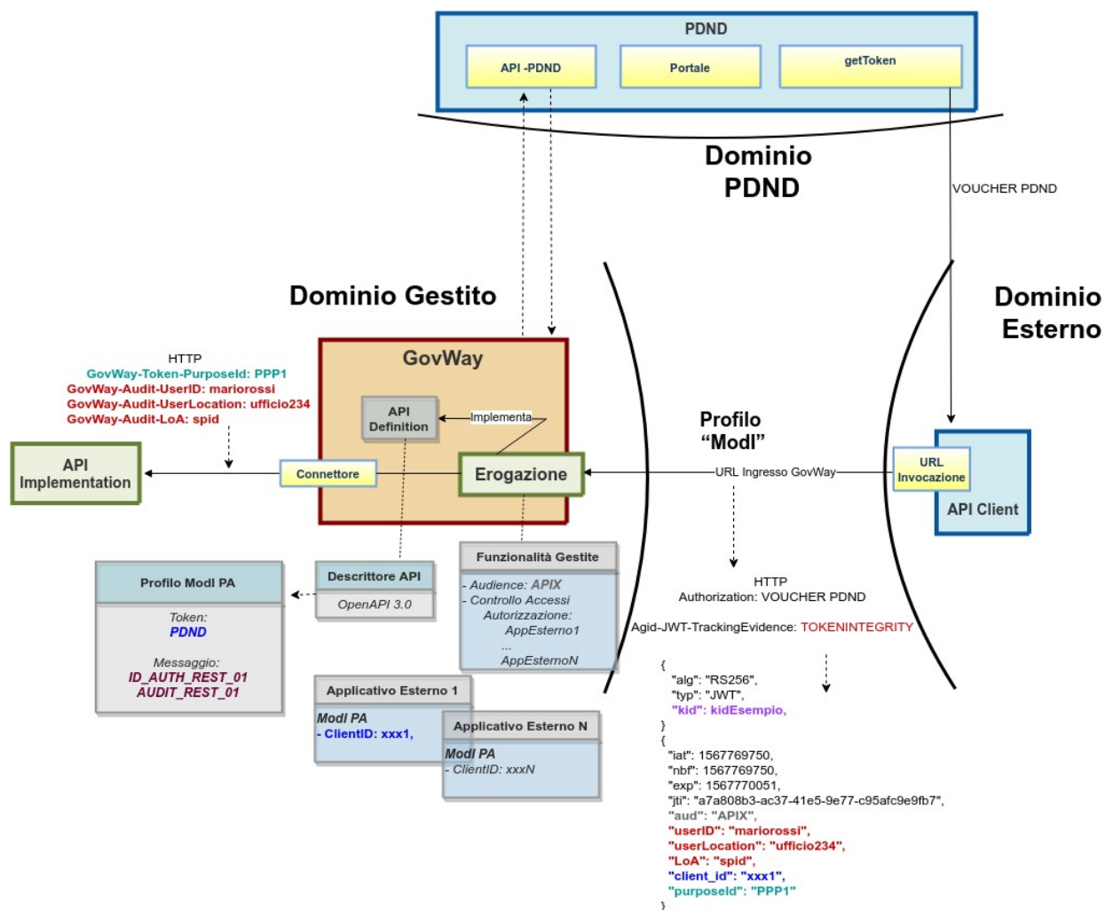
Figure3.97: Erogazione con Profilo di Interoperabilità “ModI”, pattern “AUDIT_REST_01”: trust tramite PDND
