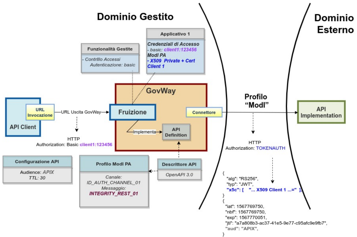
Figure3.50: Fruizione con Profilo di Interoperabilità "ModI", pattern "ID_AUTH_REST_01": trust tra fruitore ed erogatore tramite certificati x509
