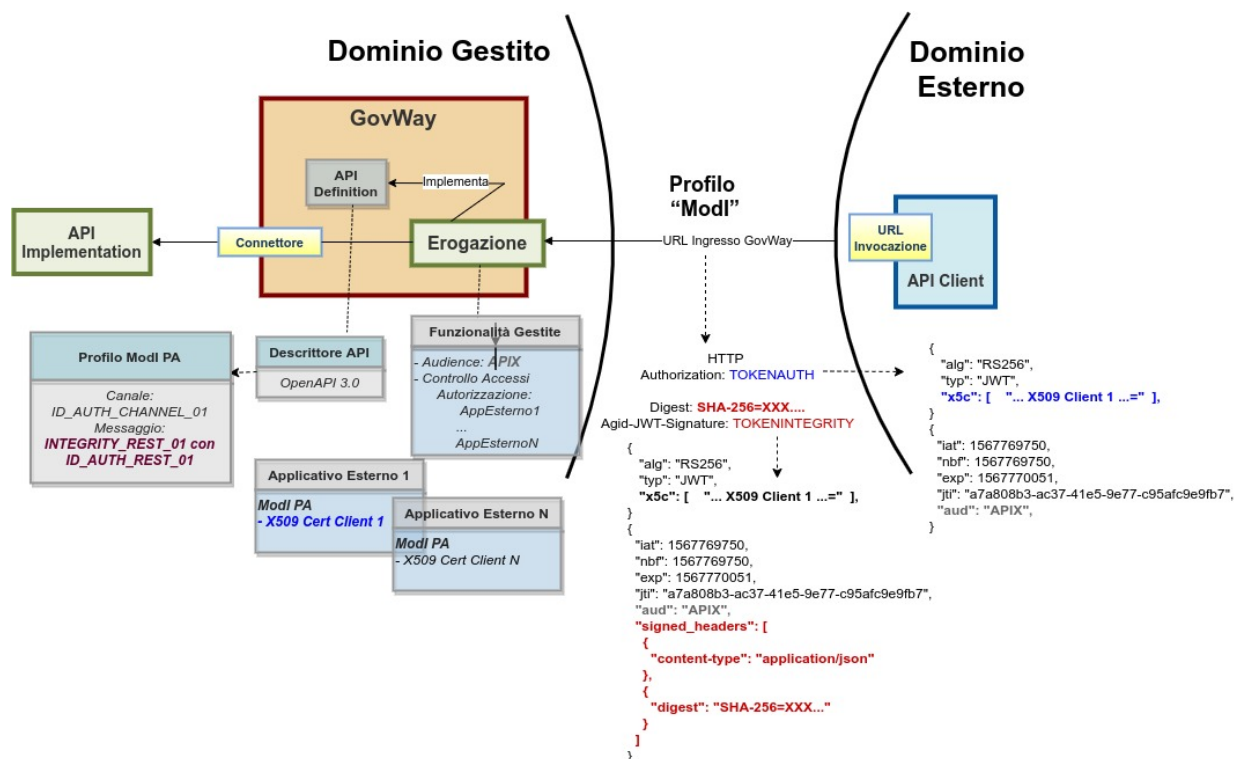
Figure3.84: Erogazione con Profilo di Interoperabilità “ModI”, pattern “INTEGRITY_REST_01”: trust tra fruitore ed erogatore tramite certificati x509
