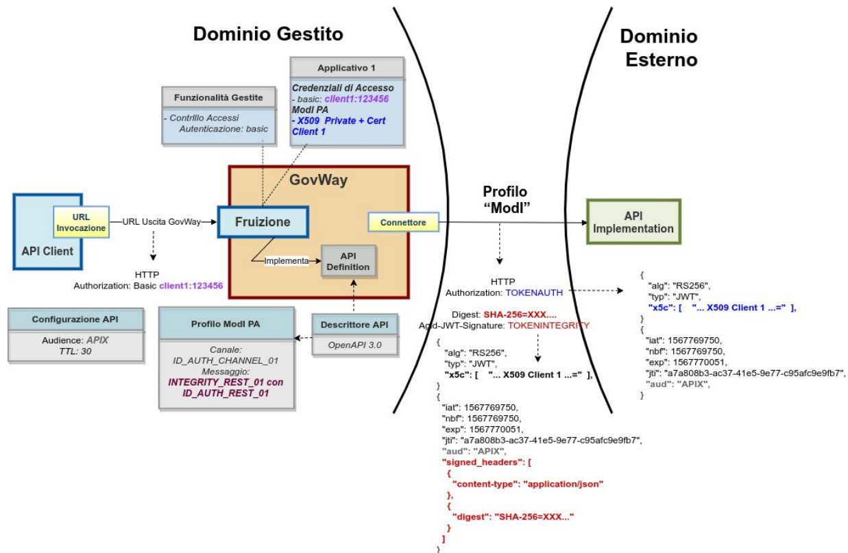
Figure3.82: Fruizione con Profilo di Interoperabilità “ModI”, pattern “INTEGRITY_REST_01”: trust tra fruitore ed erogatore tramite certificati x509
