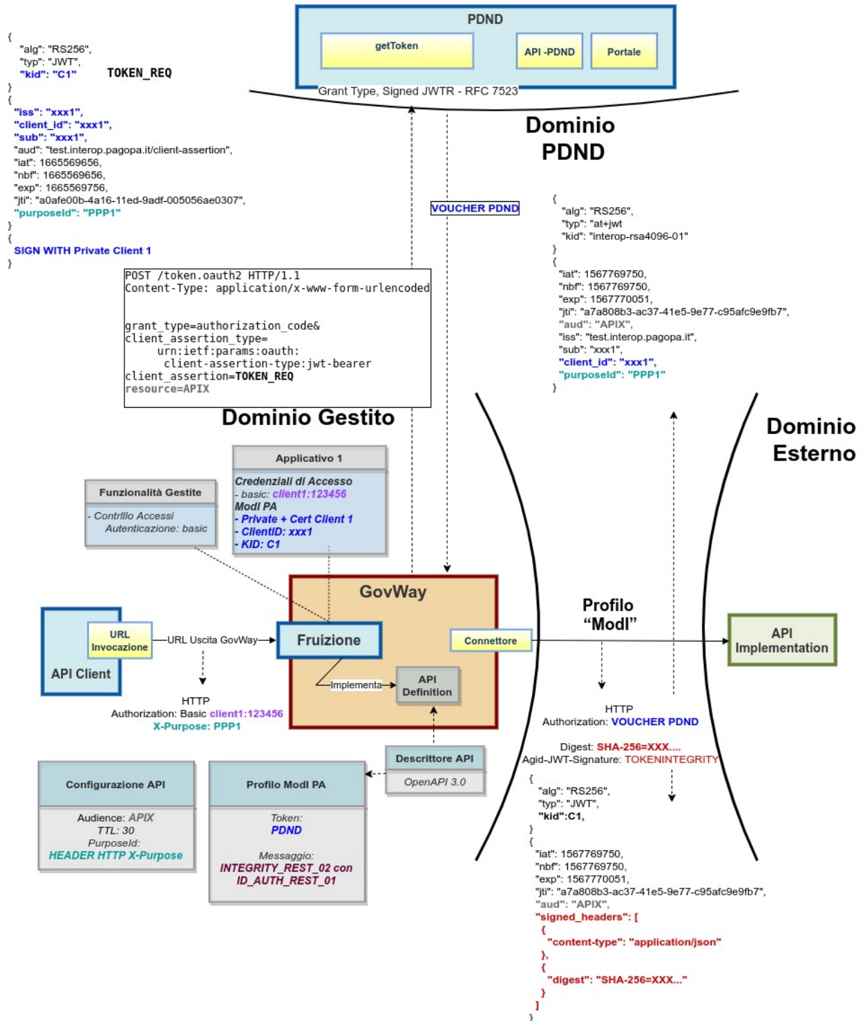
Figure3.69: Fruizione con Profilo di Interoperabilità “Modi”, pattern “INTEGRITY_REST_02”: trust tramite PDND
