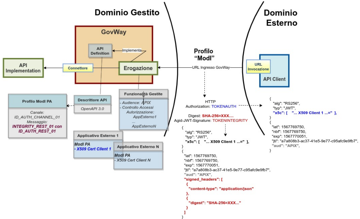
Figure3.84: Erogozione con Profilo di Interoperabilità "Modi", pattern "INTEGRITY_REST_01": trust tra fruitore ed erogatore tramite certificati x509
