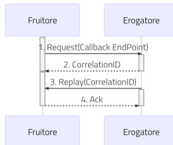
Figure3.139: Flusso previsto in un Pattern di Interazione PUSH
