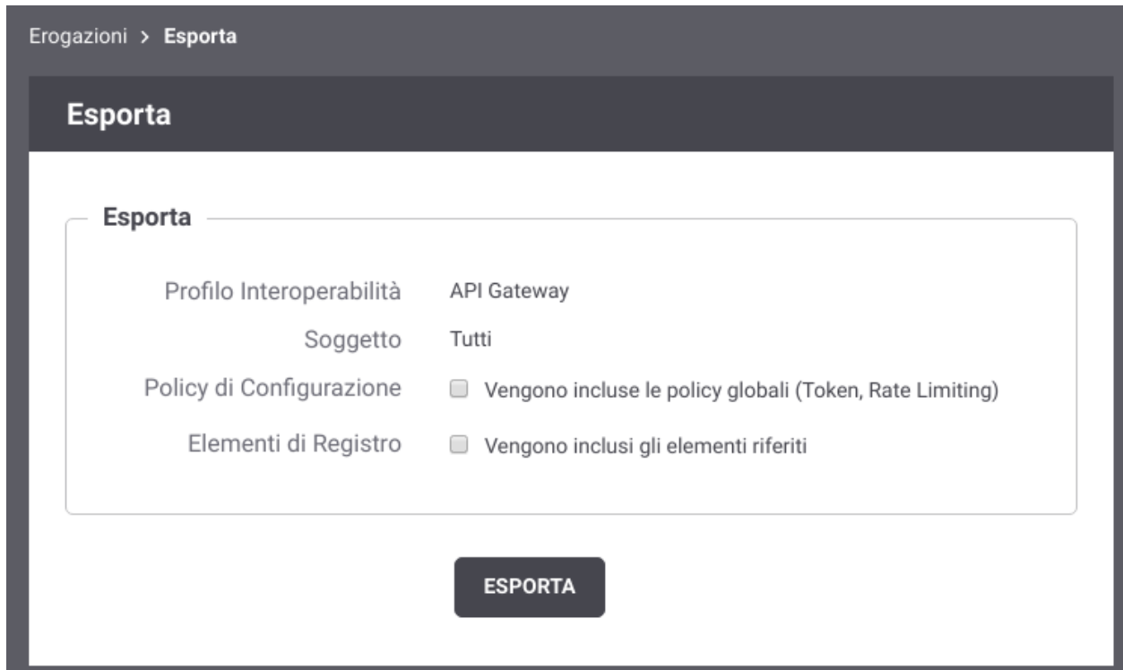
Figure8.105: Esportazione di entità nel registro: parametri
