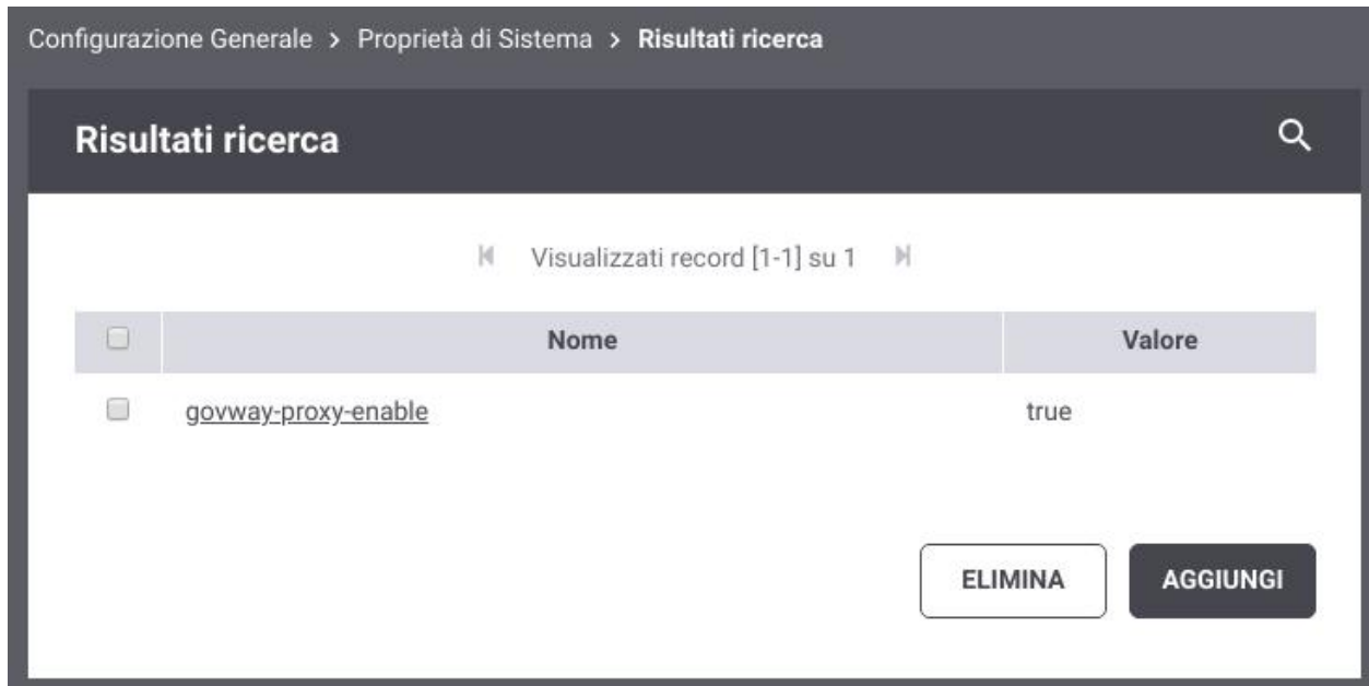
Figure10.24: Configurazione delle Proprietà di Sistema
