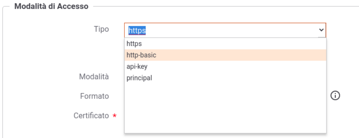
Figure2.79: Configurazione della Modalità di Accesso
