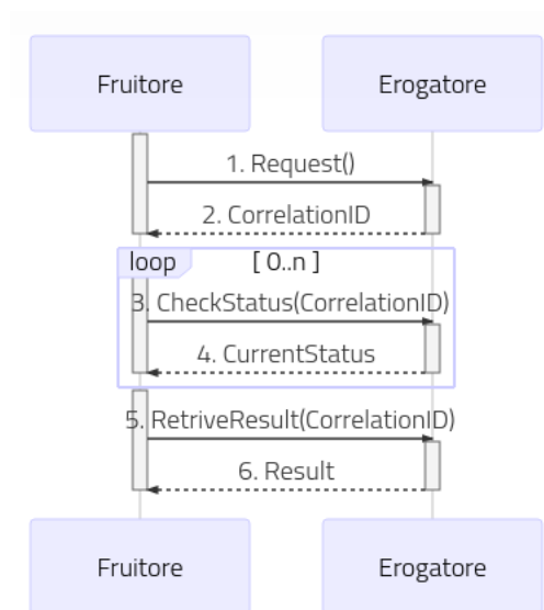
Fig. 3.137: Flusso previsto in un Pattern di Interazione PULL per API SOAP
