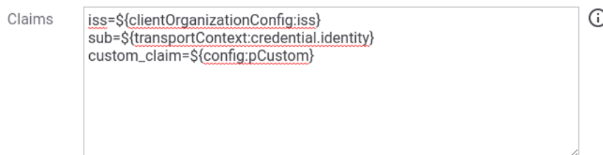
Fig. 3.118: Claims aggiuntivi inseriti nel Payload JWT
