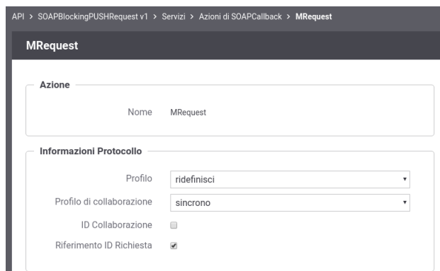
Fig. 3.131: Abilitazione funzionalità di correlazione govway tramite identificativo della richiesta
