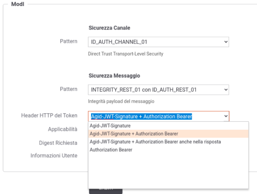
Fig. 3.110: Selezione dell'Header HTTP del token JWT
