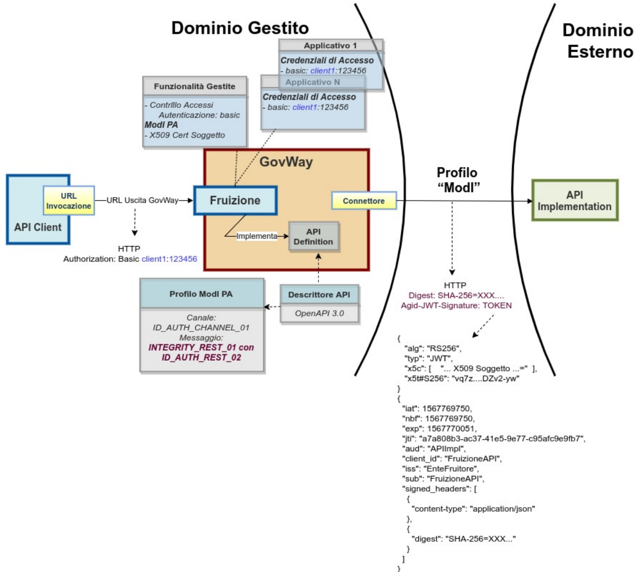
Fig. 3.122: Fruizione con Profilo di Interoperabilità "ModI"; keystore definito nella fruizione
