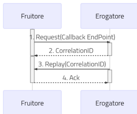
Fig. 3.127: Flusso previsto in un Pattern di Interazione PUSH
