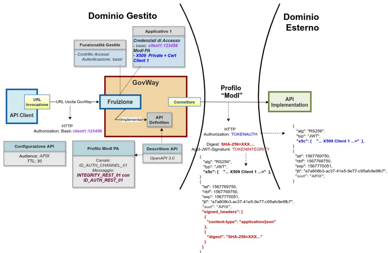
Fig. 3.82: Fruizione con Profilo di Interoperabilità “Modl”, pattern “INTEGRITY_REST_01”: trust tra fruitore ed erogatore tramite certificati x509
