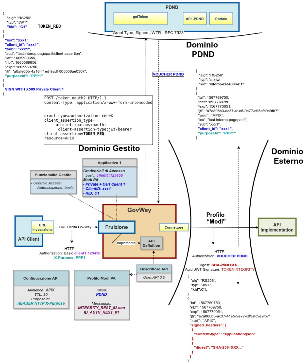
Fig. 3.7: Fruizione con Profilo di Interoperabilità “ModI”: trust tramite PDND
